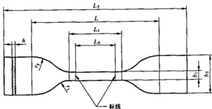
图 1 2 型试样
